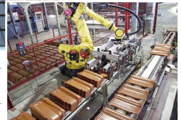
unten: Entladung der Dachziegel via Roboter.
