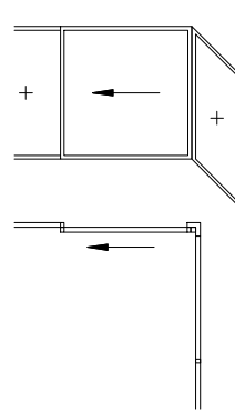
Schieber Innenecke mit Profil
