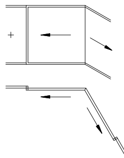
Schieber Innenecke Ganzglas "Sonder-Winkel"
