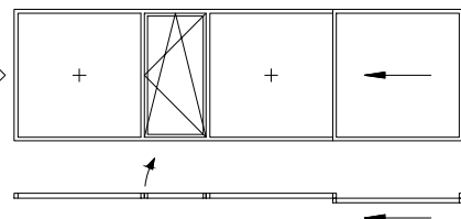
Schieber seitlich mit Festverglasung und Drehkipp-Fenster
