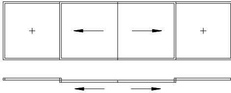
Schieber Mitte (Vertikalstoss Ganzglas)
