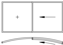
Schieber mit Festverglasung "Innenbogen"
