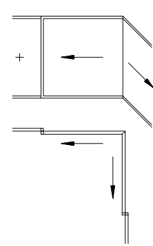
Schieber Innenecke Ganzglas
