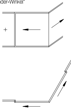
Schieber Aussenecke Ganzglas "Sonder-Winkel"
