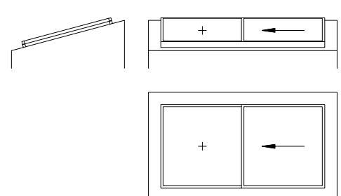
Schieber mit Festverglasung "Dach-Schieber"
