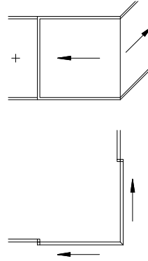
Schieber Aussenecke Ganzglas
