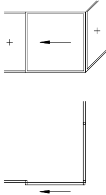
Schieber Aussenecke mit Profil
