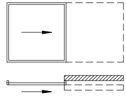
Schieber Innenecke Ganzglas
