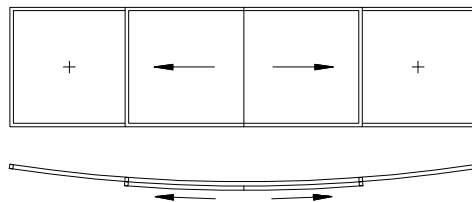
Schieber Mitte (Innenbogen) (Vertikalstoss Ganzglas)
